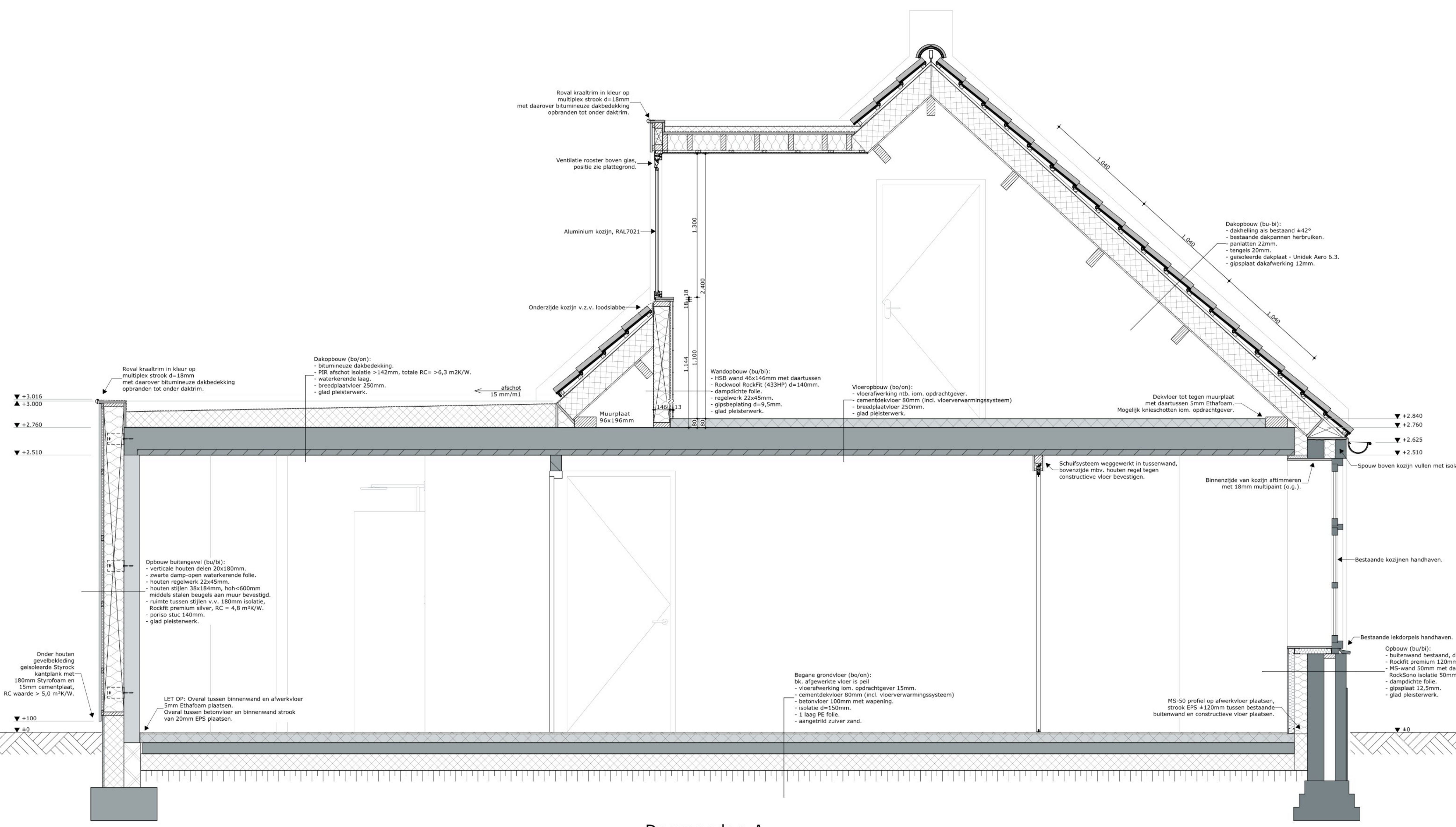
Doorsneden A
