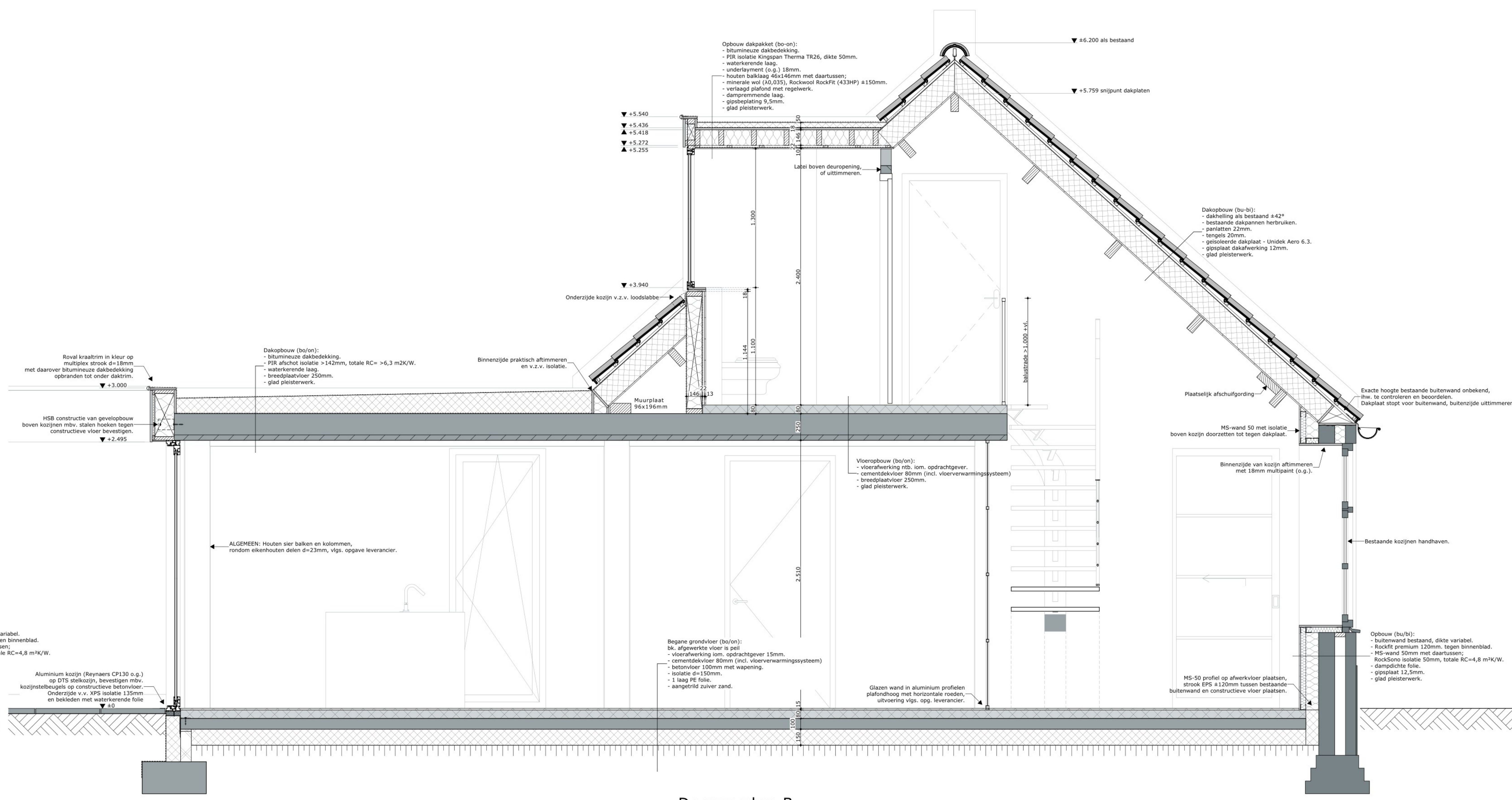
Doorsneden B
