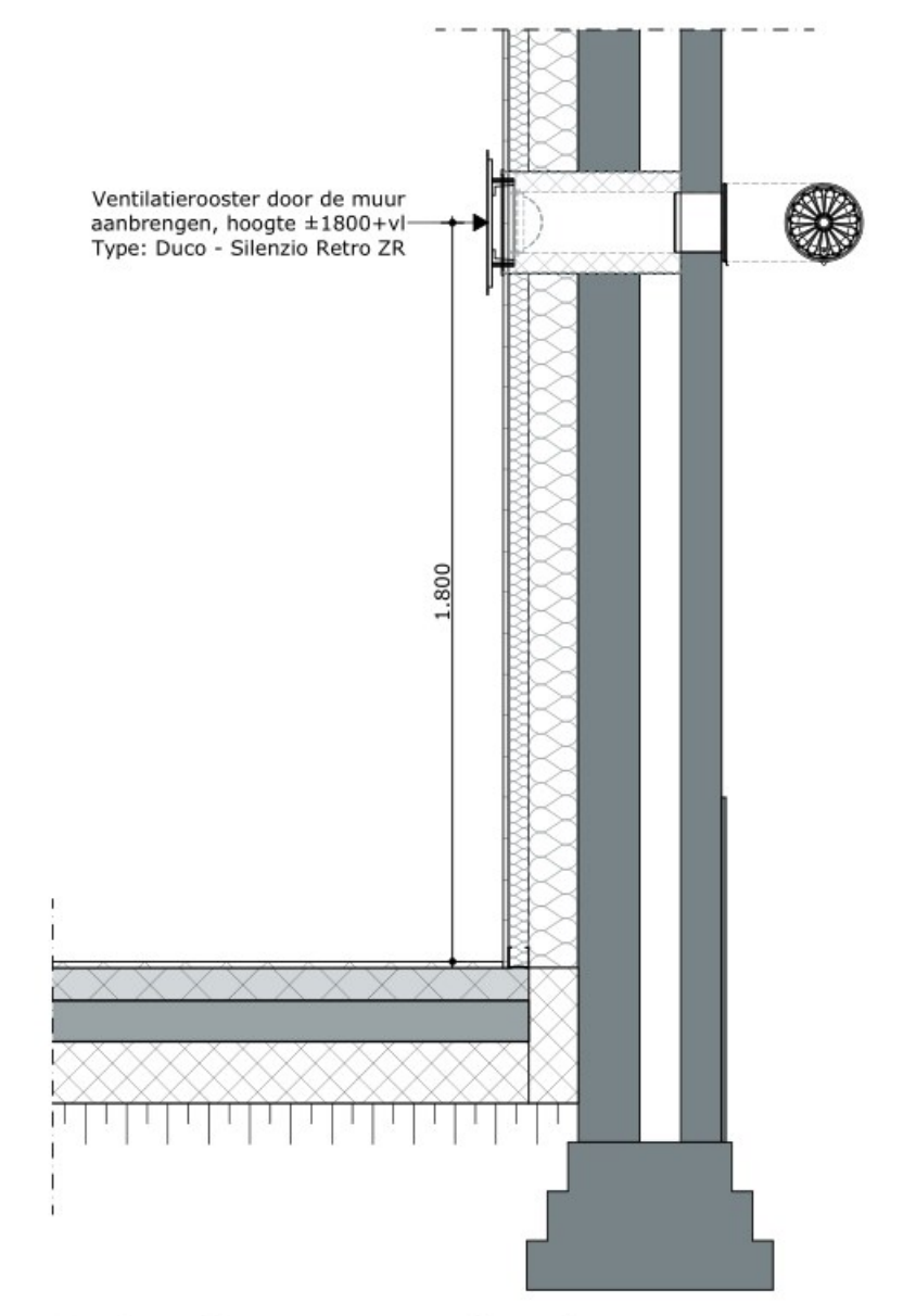
Principe ventilatie rooster door muur
